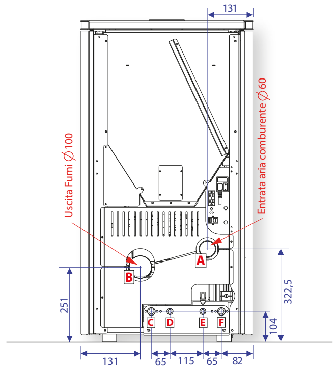
Vista Dietro
